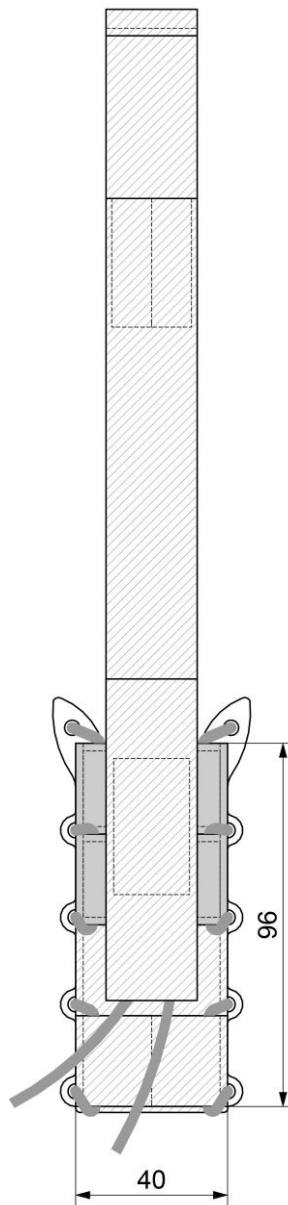
Рисунок Д1.1 – Орієнтовний зовнішній вигляд предмета (закритий)
